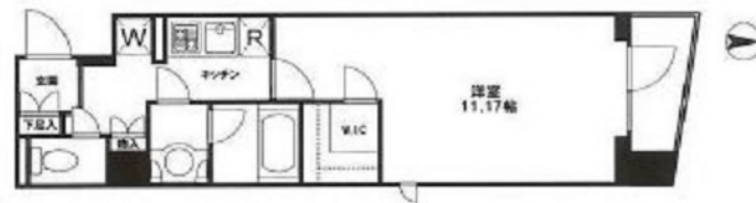
【間取り図】
